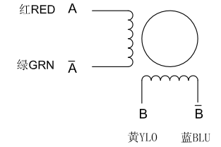
接线图 WINDING DIAGRAM
